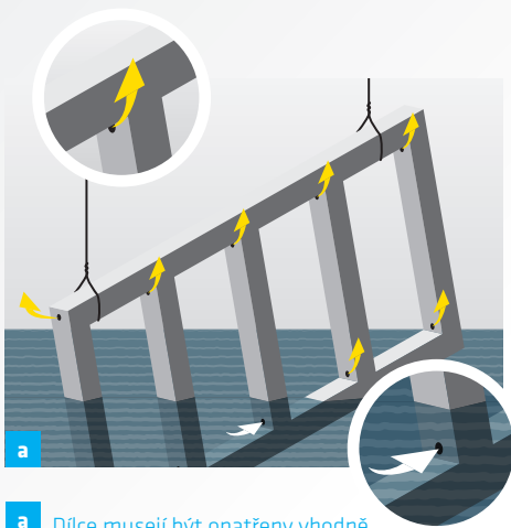
a Dílce musejí být opatřeny vhodně umístěnými a dostatečně dimenzovanými vtokovými a odtokovými otvory, jinak není zaručen optimální výsledek zinkování. Za určitých okolností může dokonce hrozit nebezpečí exploze.
