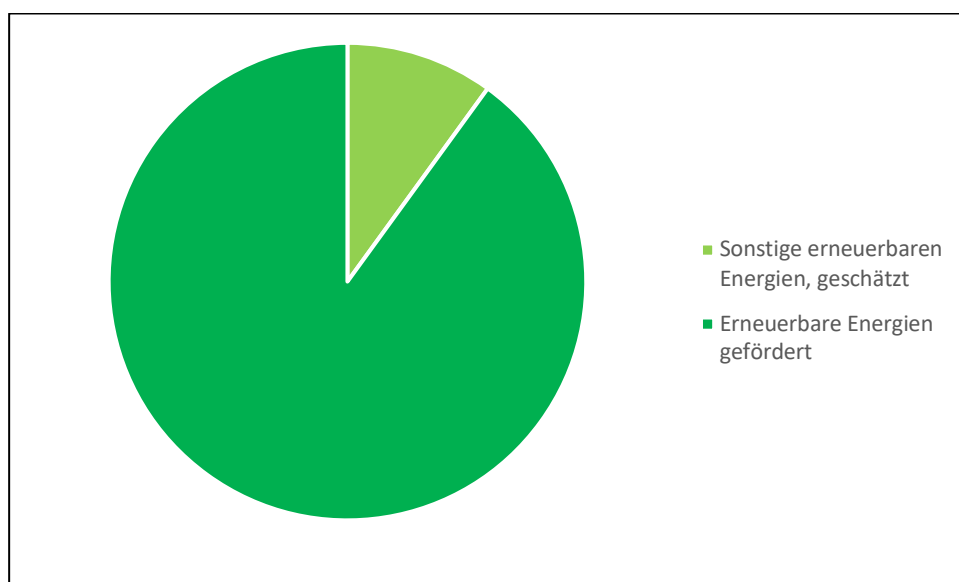
Deutscher Strommix 2025
