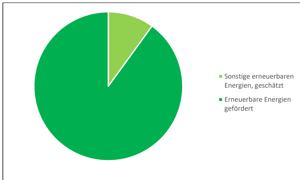
Deutscher Strommix 2022
