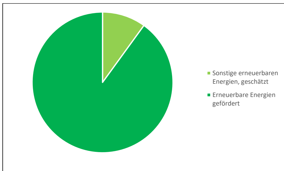
Deutscher Strommix 2022
